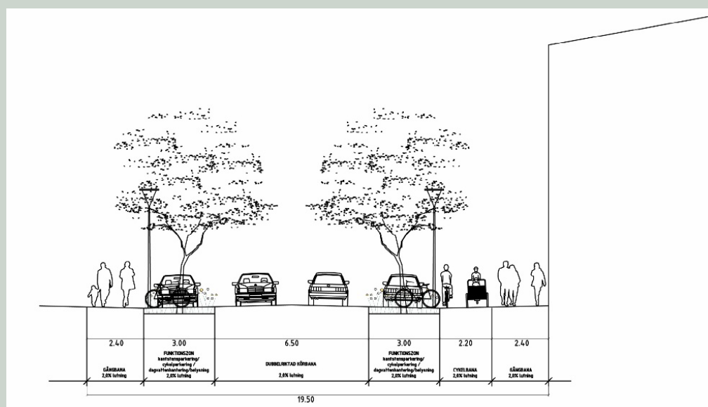
Figur: Sektion B-B som visar Cv-gatan i norr med gång- cykelbanor och funktionszoner, Tengbom
