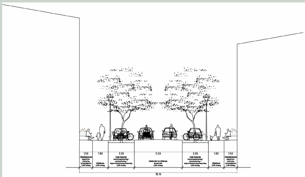
Figur: Sektion A-A som visar gata i väster med gång- cykelbanor och funktionszoner, Tengbom
