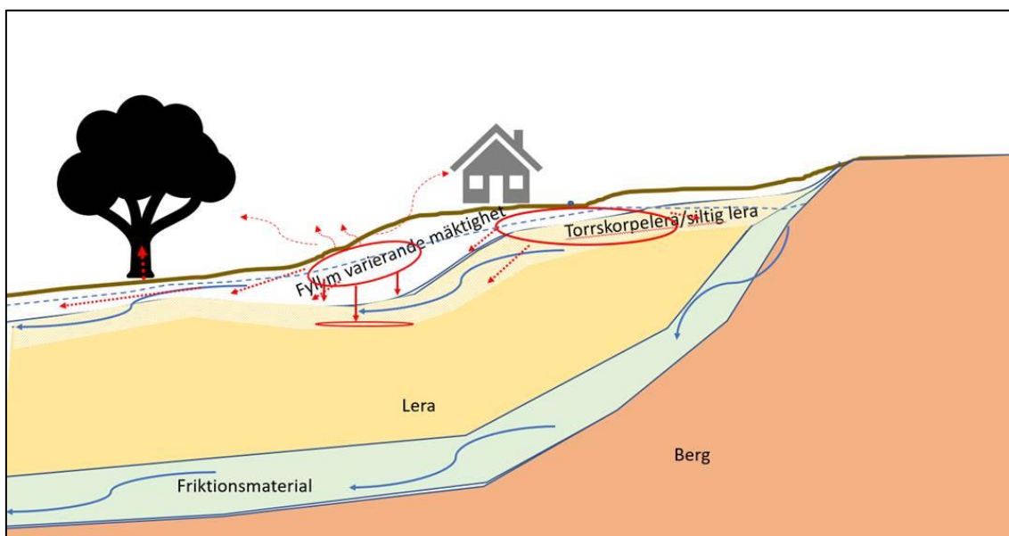
Figur 3. Konceptuell modell avseende geologi och hydrogeologi inom CV-området, Etapp 1.
