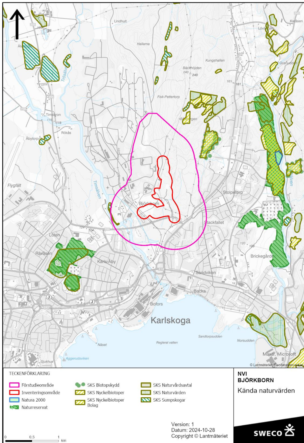
Figur 5. Omgivande kända naturvärden.
