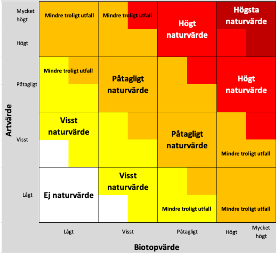
Figur 1. Schematisk matris enligt standard för bedömning av naturvärden baserat på art- respektive biotopvärde. Bild från SS 199000:2023.
